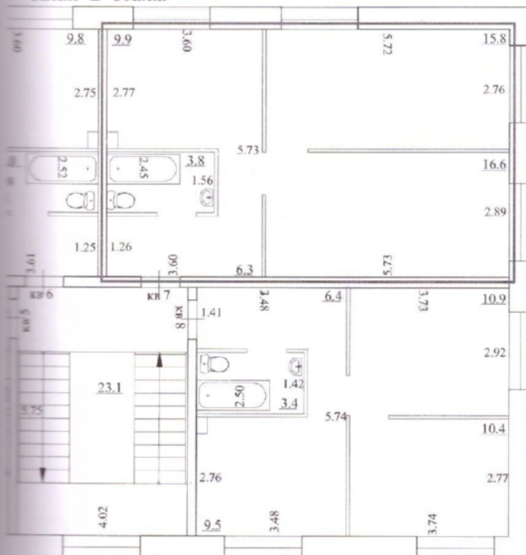
План 2 этажа
