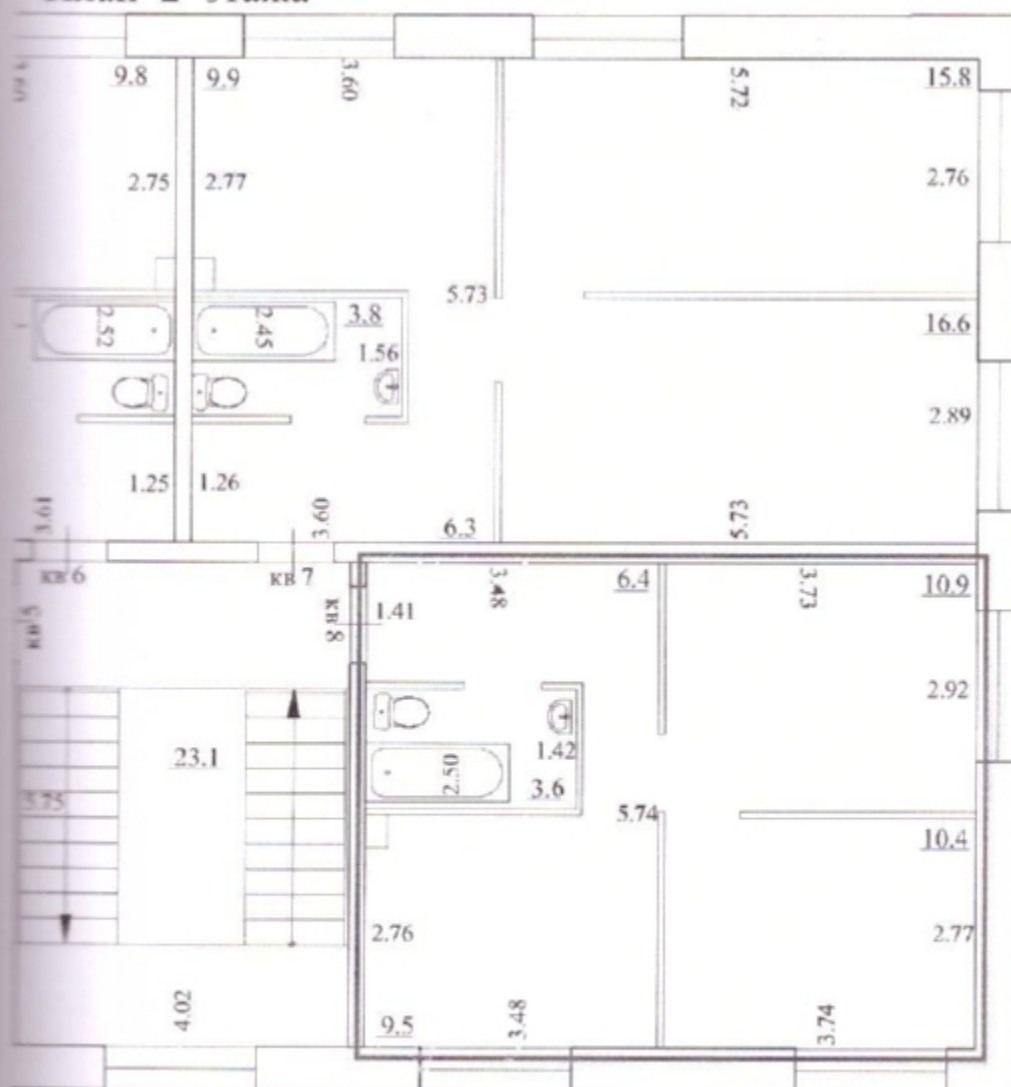
План 2 этажа
