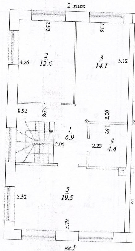
Экспликация помещений 2 этаж :
